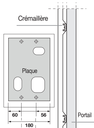
ANCRAGE DU MOTORÉDUCTEUR vue en plan
