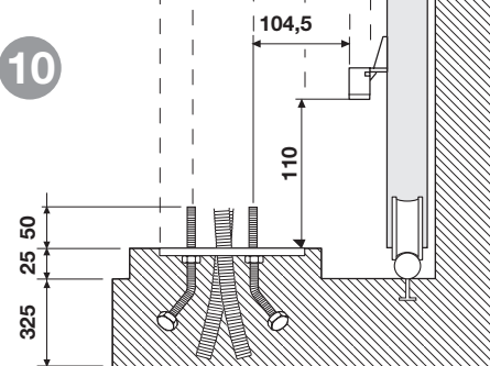
ANCRAGE DU MOTORÉDUCTEUR vue latérale
