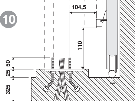
ANCLAJE Vista lateral
